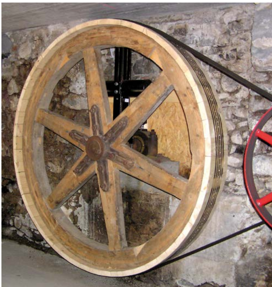
Altes Antriebsrad mit neuem Riemenkranz
