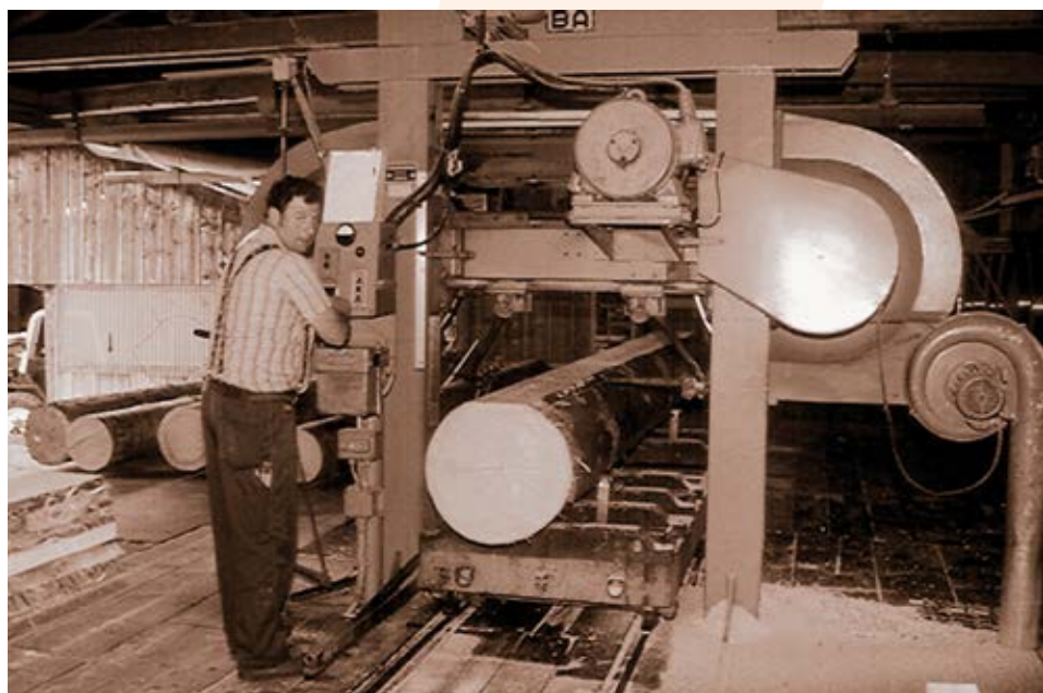
Elektrisch betriebene Horizontalblockbandsäge mit dem letzten Säger
